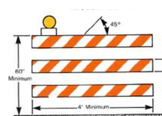
Type III Barricade
