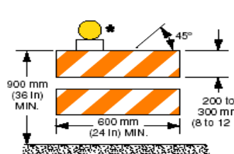
Type II Barricade
