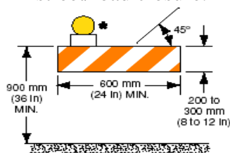
Type I Barricade
